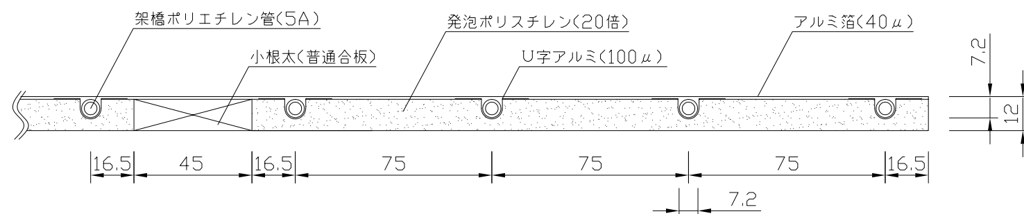
(A-A'断面図)
