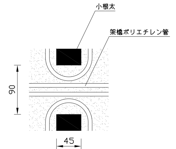
(小根太-小根太間拡大図)
